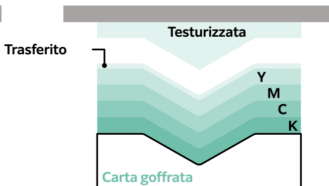
Nastro di trasferimento intermedio
