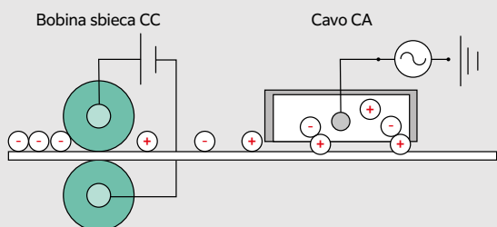
Eliminatore dell'elettricità statica
