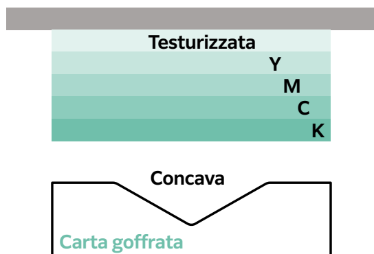
Nastro di trasferimento intermedio
